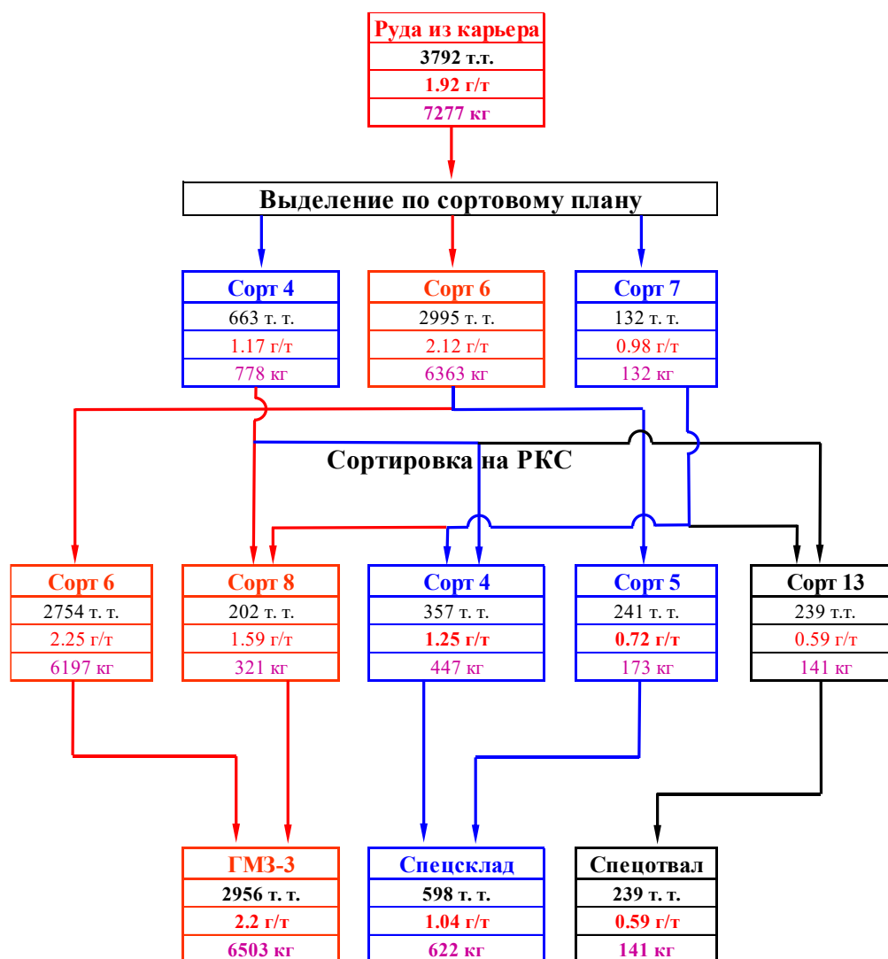
Рисунок 7 Качественно-количественная схема предварительного обогащения золото - сульфидных руд, на РКС месторождения Кокпатас.
