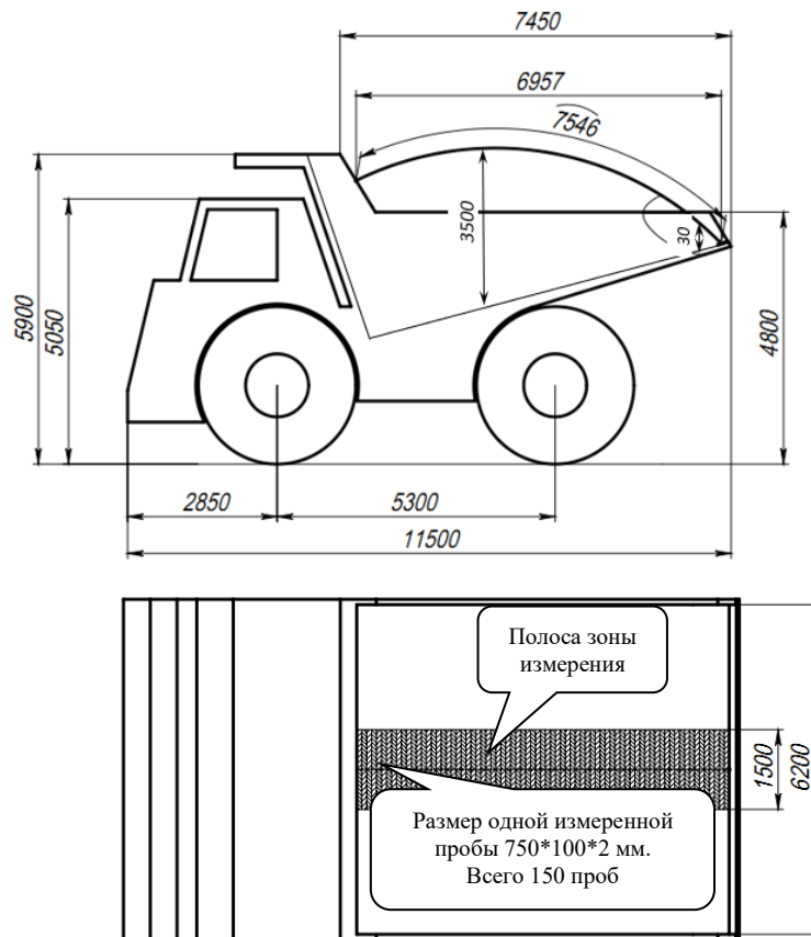
Рисунок 2 Параметры кузова и зоны измерения руды в Белазе - 7513
