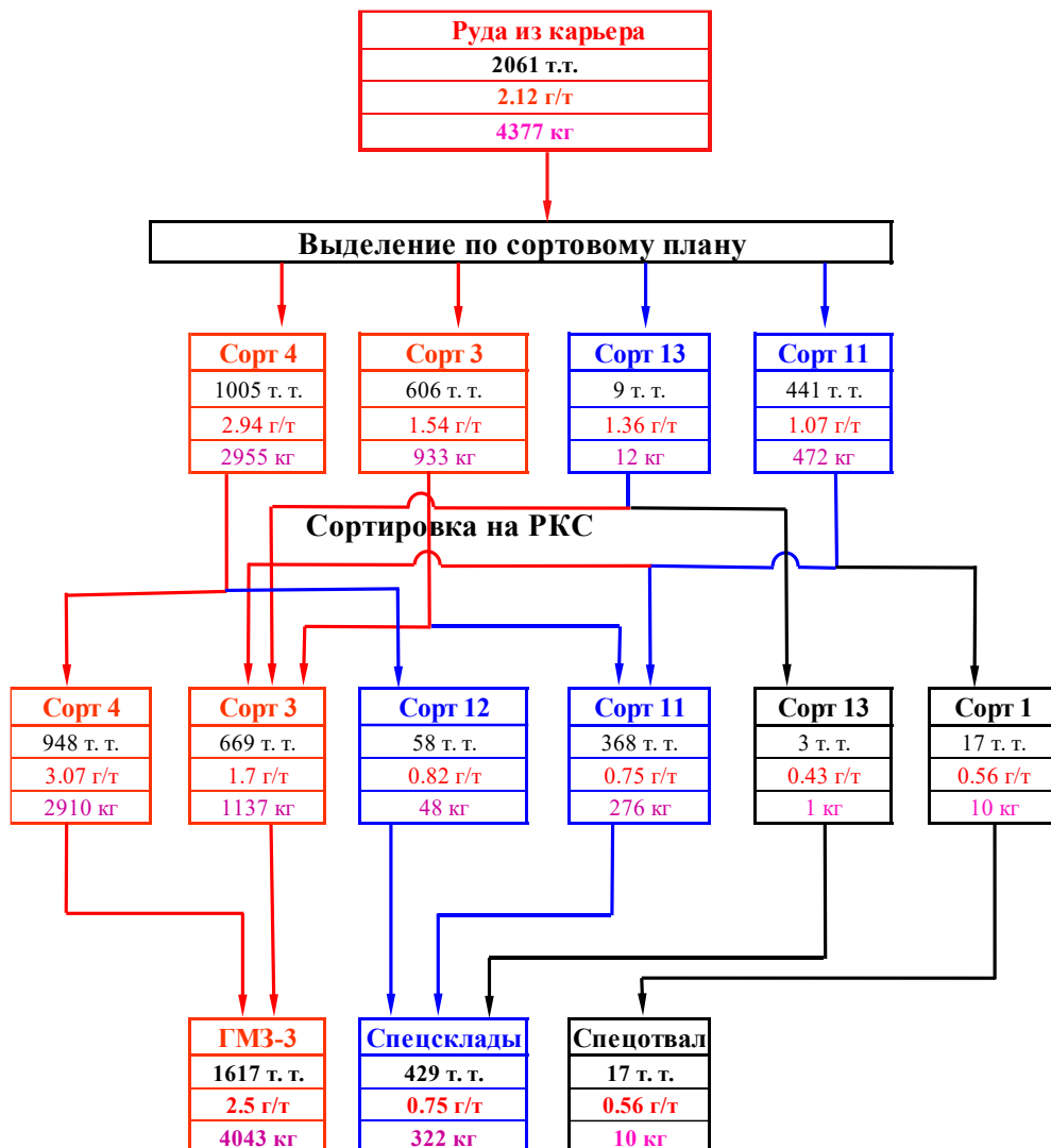
Рисунок 10 Качественно-количественная схема предварительного обогащения золото - сульфидных руд, на РКС месторождения Даугызтау.
