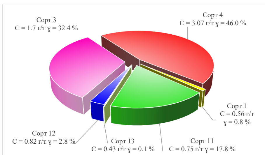
Рисунок 8 Диаграмм соотношения объемов и содержаний выделенных сортов руд на РКС месторождения Даугызтау.
