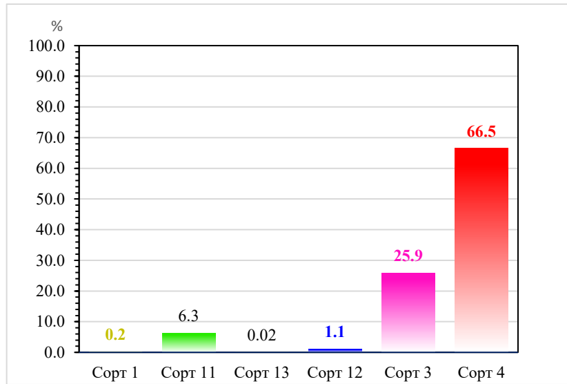
Рисунок 9 Количество металла в %, в выделенных сортах руд на РКС месторождения Даугызтау.
