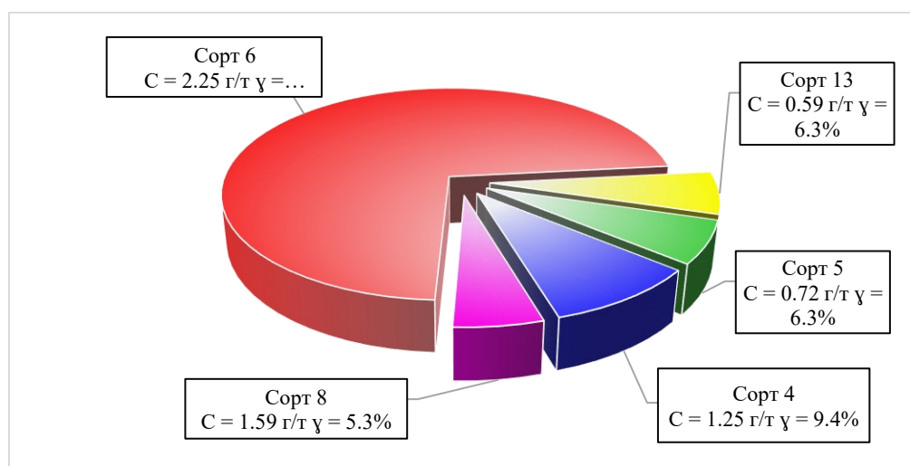
Рисунок 5 Диаграмма соотношения объёмов и содержаний выделенных сортов руд на РКС месторождения Кокпатас.
