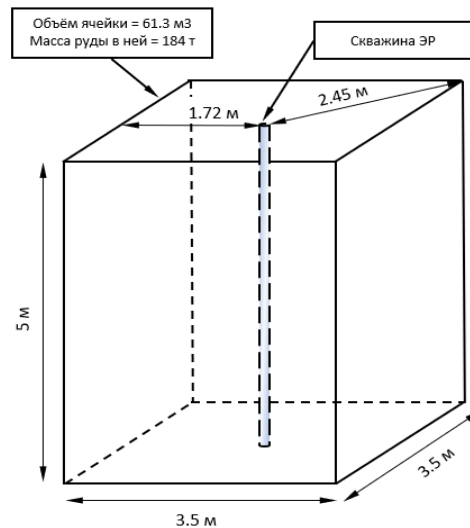
Рис 1 Размеры ячейки руды в недрах, опробываемой одной скважиной эксплуатационной разведки.
