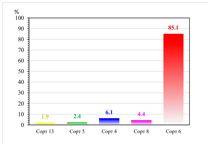
Рисунок 6 Количество металла в %, в выделенных сортах руд на РКС месторождения Кокпатас.
